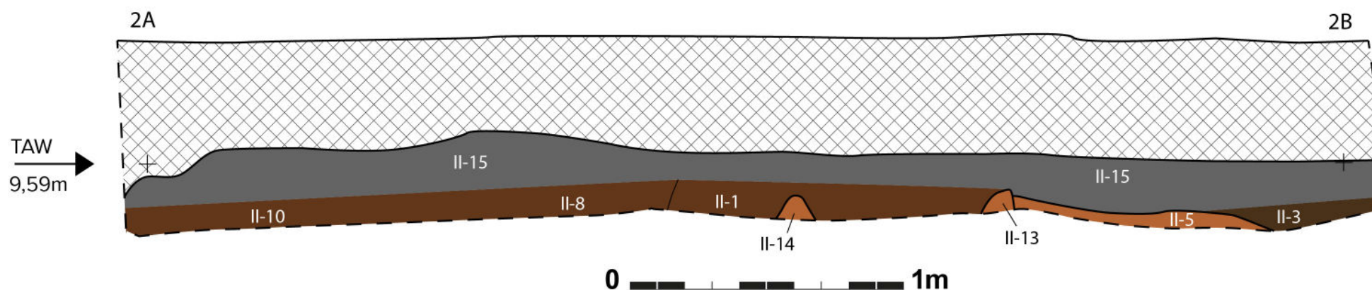
Afbeelding 2: Profiel 2AB.
