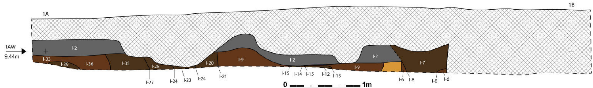
Afbeelding 1: Profiel 1AB.
